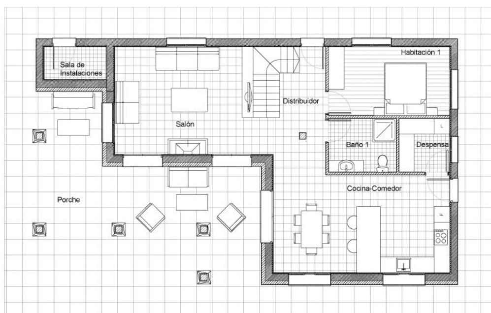
Planta baja Escala 1/100
