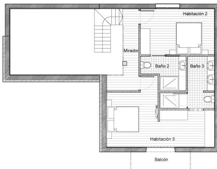
Planta primera Escala 1/100
